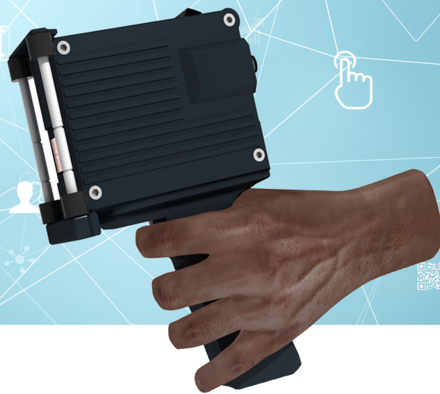
DK Mini Mobile (encoder with 4 wheels))
